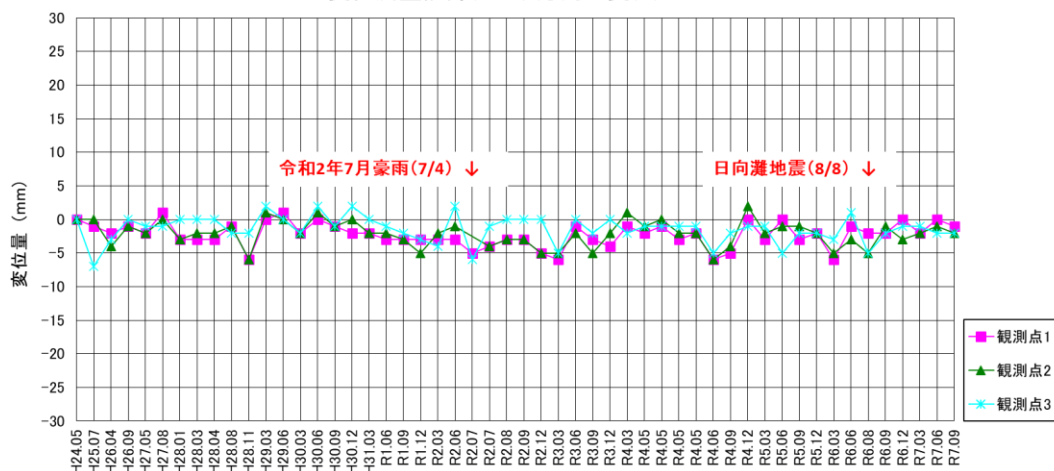
変位測量記録(上・下方向の変化)
