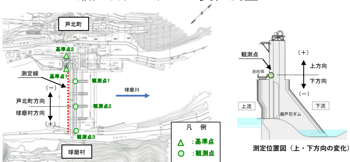
変位測量記録(上・下方向の変化)
