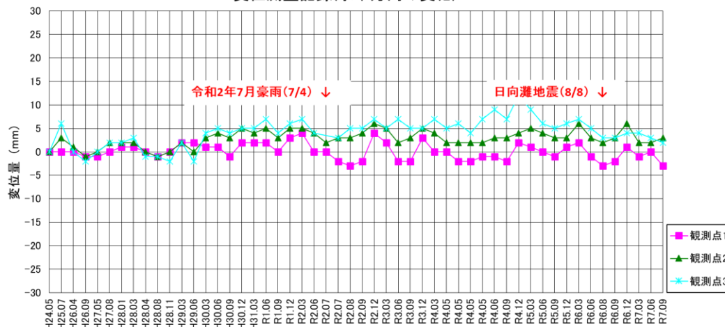
変位測量記録(水平方向の変化)
