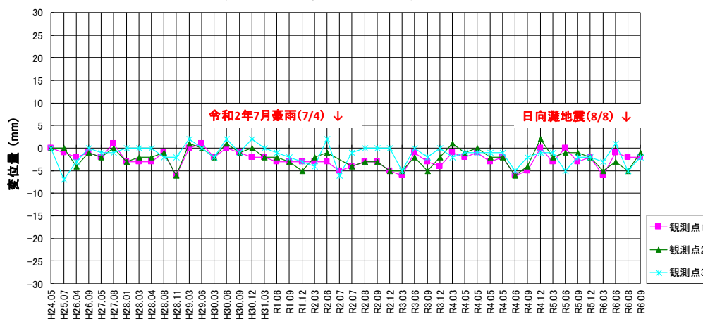
変位測量記録(上・下方向の変化)
