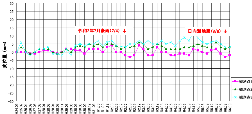
変位測量記録(水平方向の変化)
