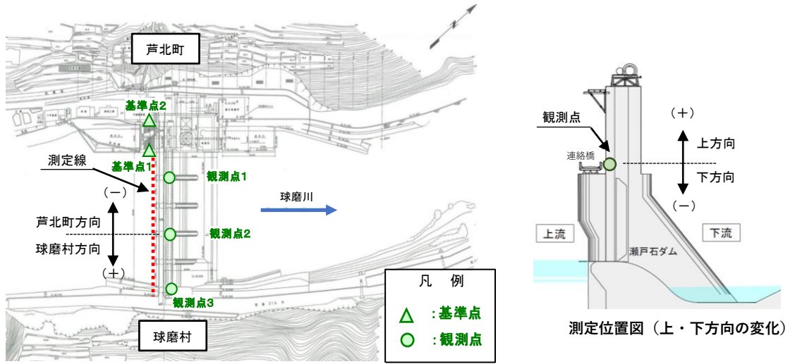
測定位置図（水平方向の変化）
