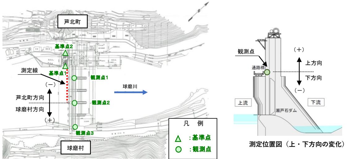
測定位置図 (水平方向の変化)
