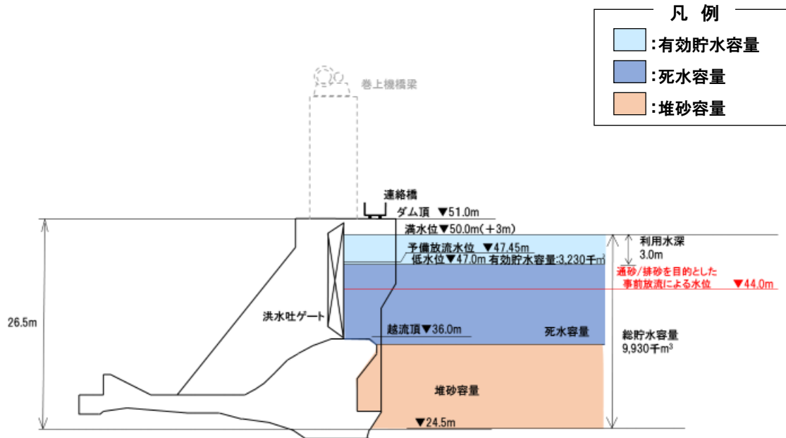
瀬戸石ダム 断面イメージ
