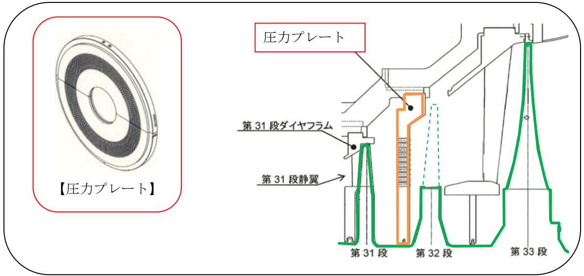
【圧カプレートの据付位置図】
