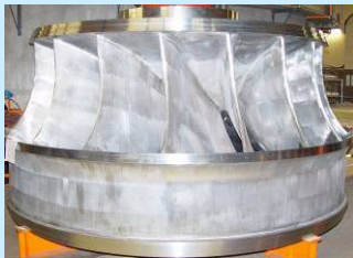
田子倉 水車ランナ
