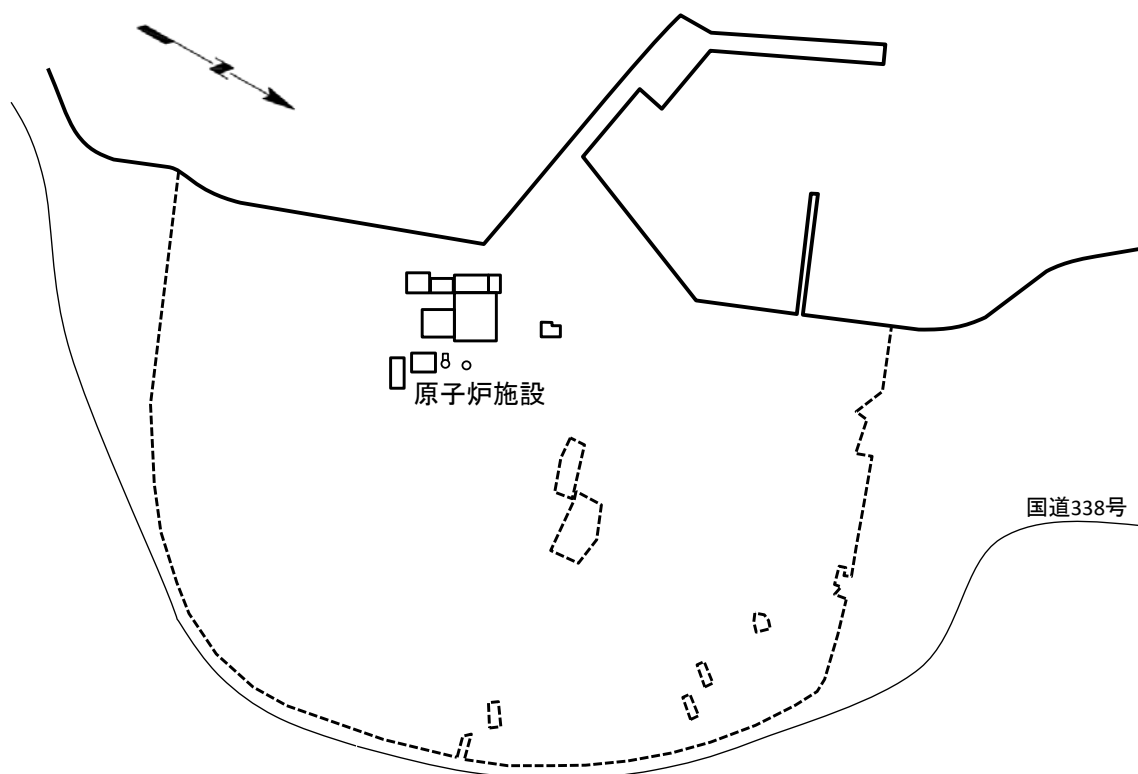
図4-1 大間原子力発電所の敷地付近の概略地図
