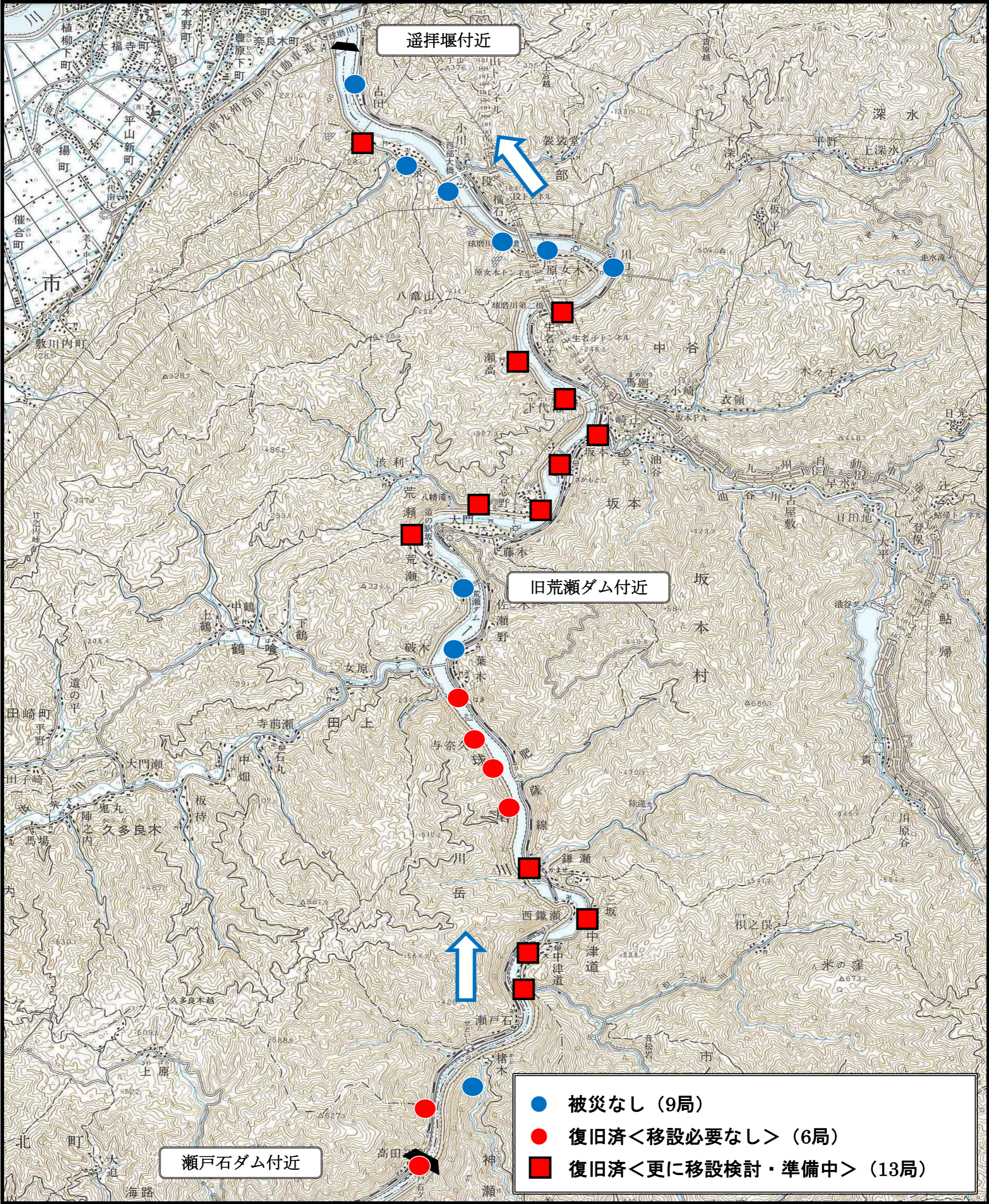
警報設備の位置及び状況図
