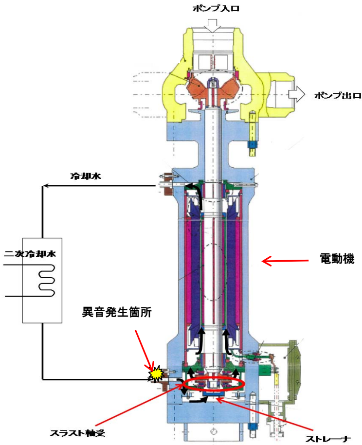
【構造図】
