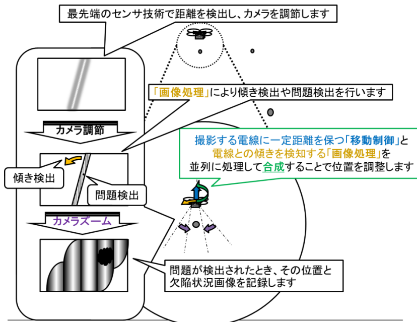
図2 画像取得技術の概要
